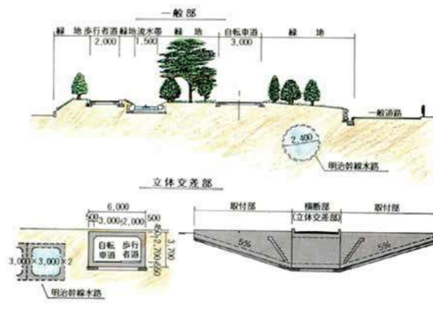
県道豊田安城自動車道線標準横断面図
